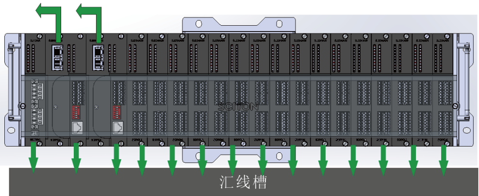
接线之前，先将加固型PLC的翻盖拆下来 由于IO模块复用了之前的PCBA，因此，接线方式仍然和之前一样，采用接插件的方式进行接线
